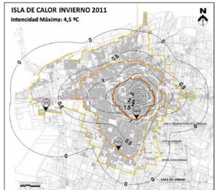
Figura 2. Isla de calor invierno del AMSJ, obtenida con procesamiento de imágenes satelitales en 2011. Fuente: Cúnsulo et al. (2013:5).
