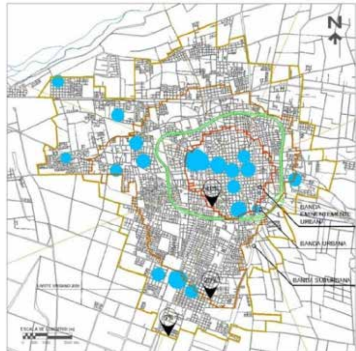
Figura 5. Cobertura térmica y húmeda del AMSJ. Fuente: Kurbán et al. (2010:10).
