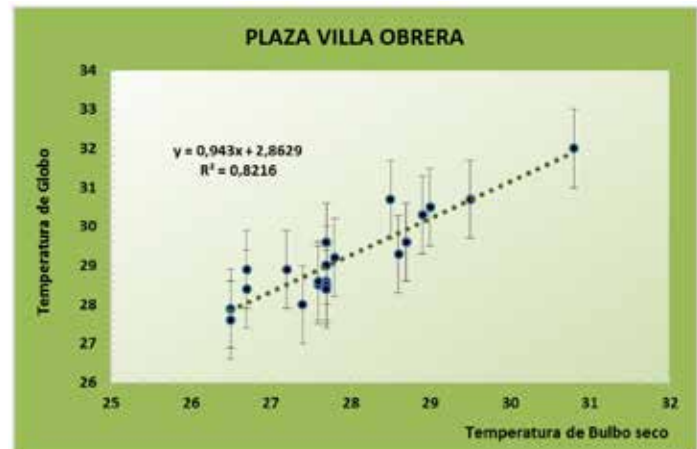
Figura 6. Correlación temperatura bulbo seco-temperatura de globo. Plaza Vª Obrera. Fuente: Elaboración de los autores.
