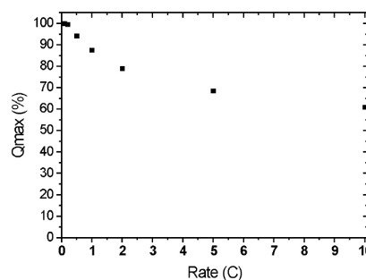
Figura 11. Capacidad de descarga en función de la velocidad de descarga.
