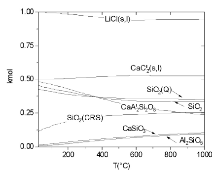
Figura 1. Composición de equilibrio del sistema Si-Al-Li-O-Ca-Cl en función de la temperatura.
