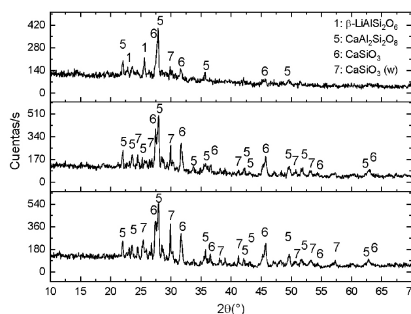
Figura 5. Patrón de difracción de la muestra clorada a 800 °C durante (a) 30 min, (b) 75 min y (c) 120 min.
