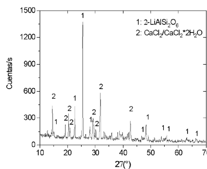
Figura 2. Patrón de DRX de la mezcla \beta\text{-LiAlSi}_2\text{O}_6/\text{CaCl}_2
