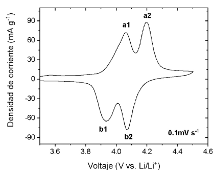
Figura 10. Voltamperograma cíclico de la espinela a temperatura ambiente.
