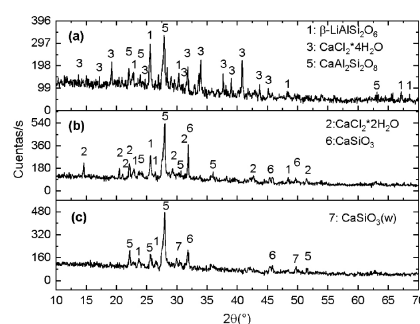
Figura 4. Patrón de difracción de la muestra clorada a 700 °C durante (a) 30 min, (b) 75 min y (c) 120 min.
