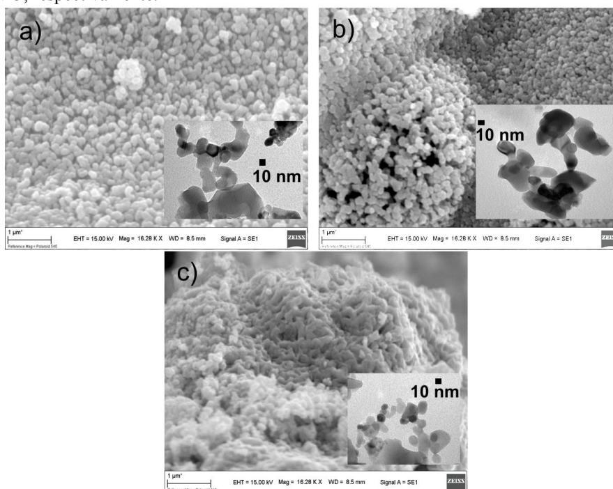
Fig. 2. Imágenes MEB y TEM de nanoestructuras de a) NiO, b) NiO-CB y c) NiO-CBf.
