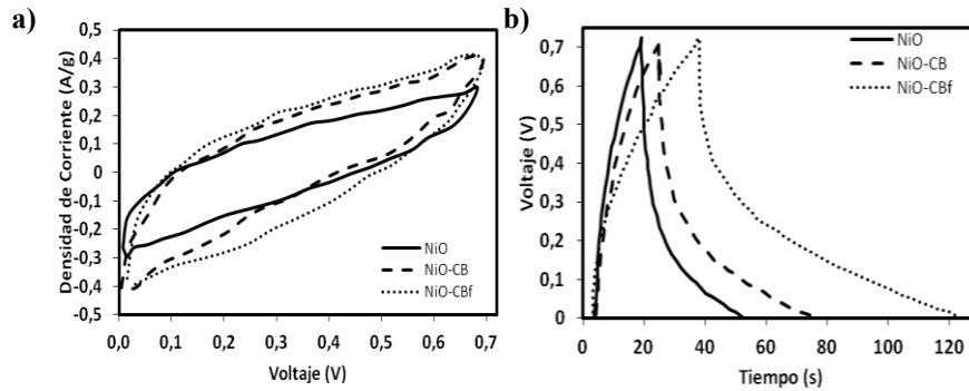
Fig. 3. a) Voltamperometría cíclica a 10 mV/s. b) Curvas galvanostáticas de carga/descarga a 3 A/g, de los nanocompuestos en KOH 1M.
