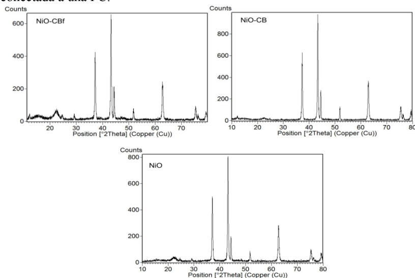
Fig. 1. Difracción de Rayos X de nanoestructuras de NiO, NiO-CB y NiO-CBf.
